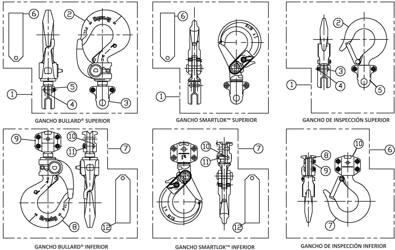
Figura 9-6 Ganchos Bullard®, SmartLok™ e Inspección
