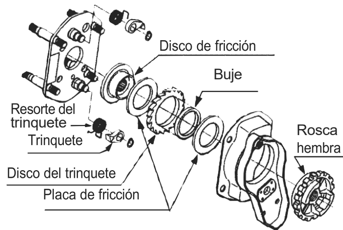
Figura 5-3 Componentes del sistema de frenos
