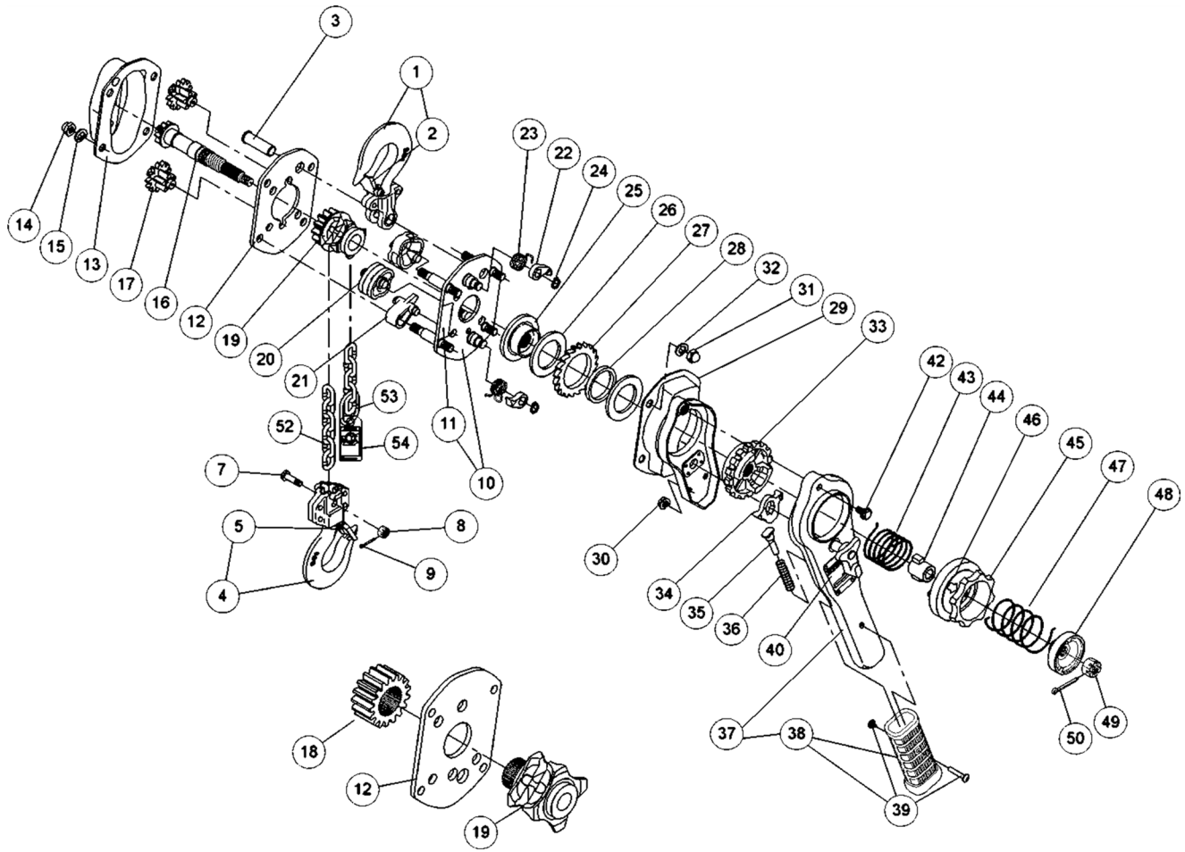
Figura 9-3 Partes para los modelos con capacidades de 0.8 a 3.2 toneladas
