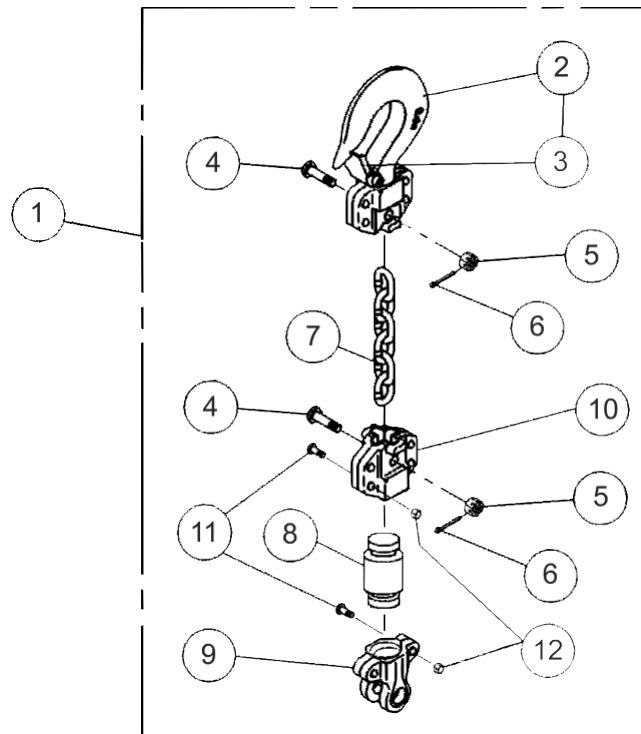
Figura 9-8 Dispositivo de extensión del gancho superior
