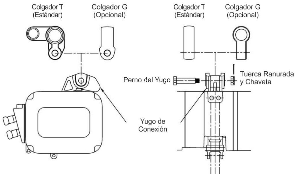
Figura 3-4 Instalación del suspensor T o G en polipastos/tecle de cadena ER2/NER2 de 2 toneladas (020C), 3 toneladas (030C) y 5 toneladas
