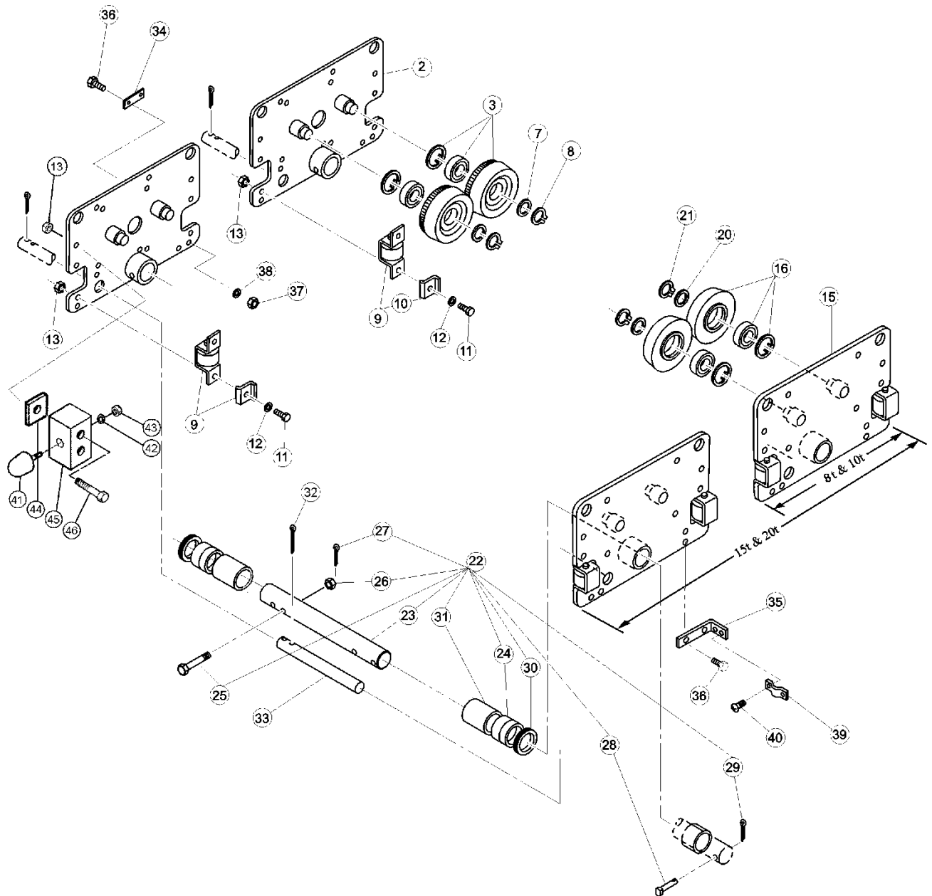
Figure 9-7 Placas Laterales y Partes de Suspensión
