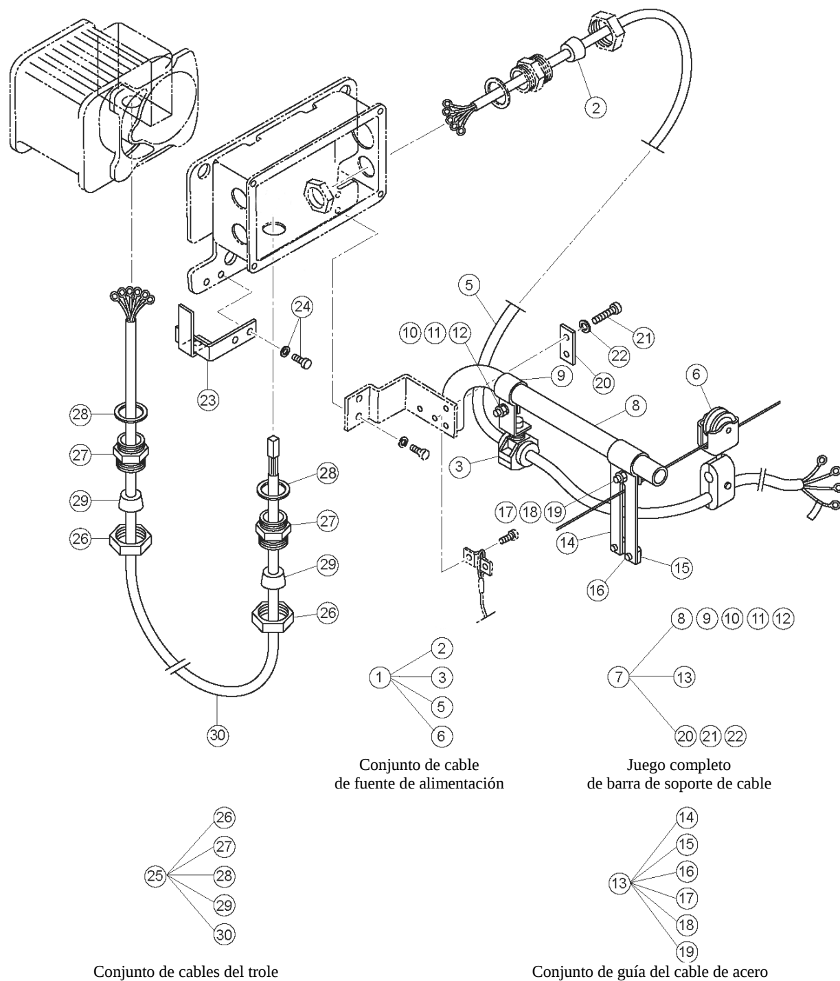
Figura 3-1 Partes de la fuente de alimentación
