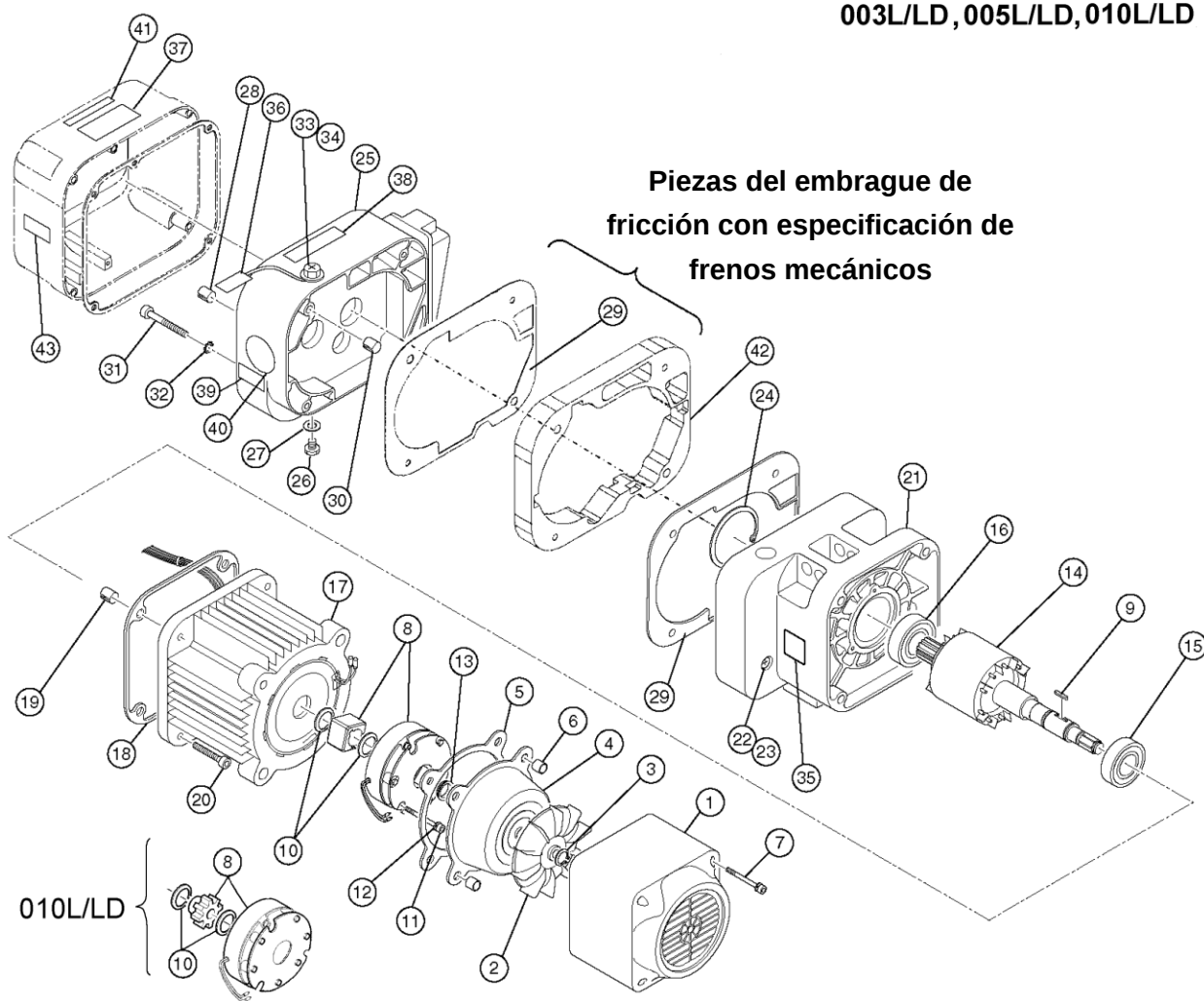
Figura 1-1 Partes del motor y de la carcasa
