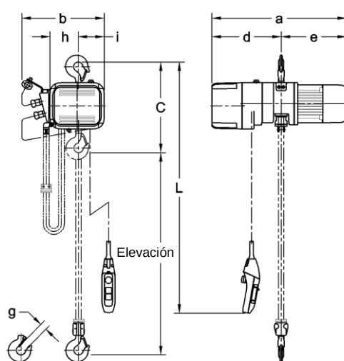
Figura 2-2 Dimensiones del polipasto/tecle de dos velocidades
