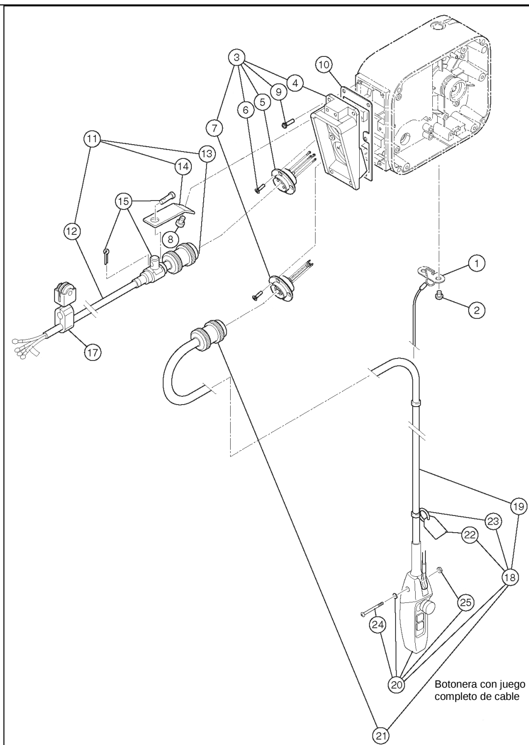
Figura 6-1 Partes de la fuente de alimentación y la botonera (conexión de enchufe)
