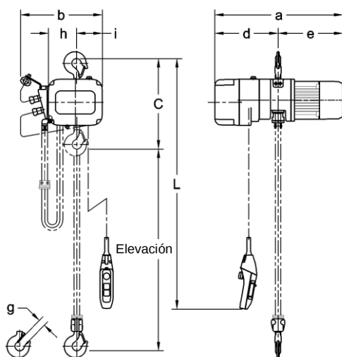
Figura 2-1 Dimensiones del polipasto/tecle de una velocidad
