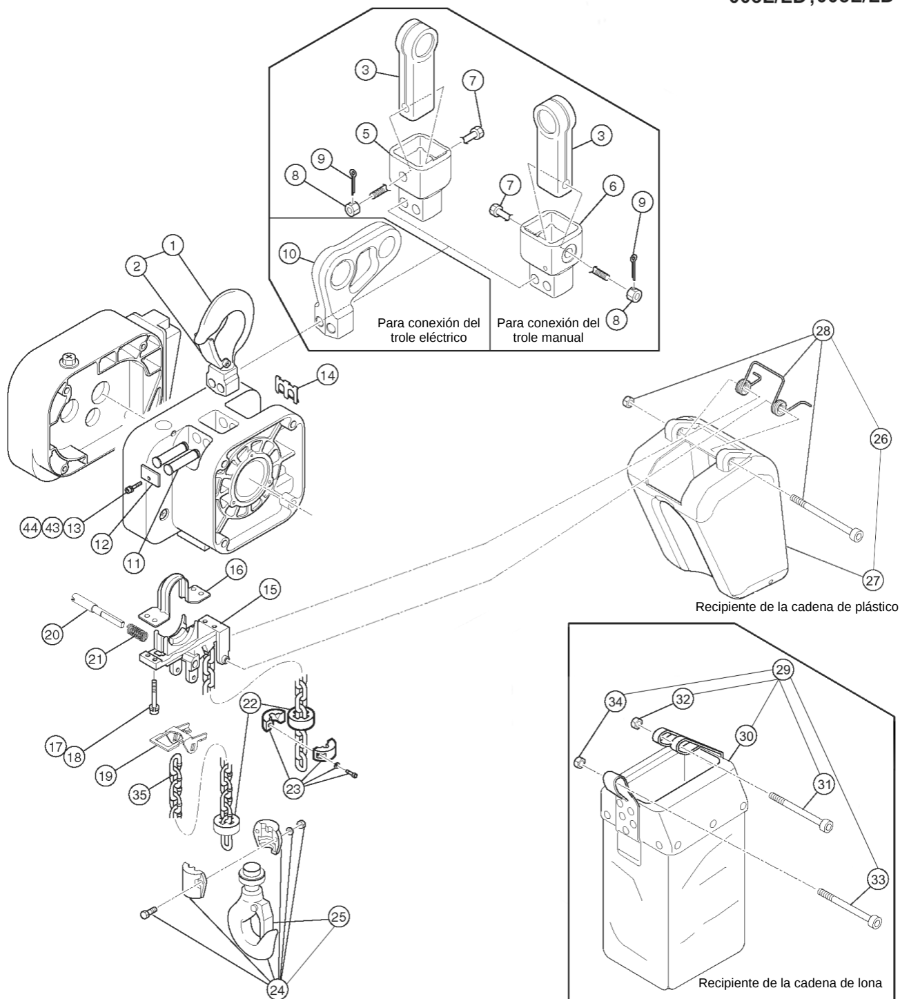
Figura 3-1 Partes del gancho y de la cadena
