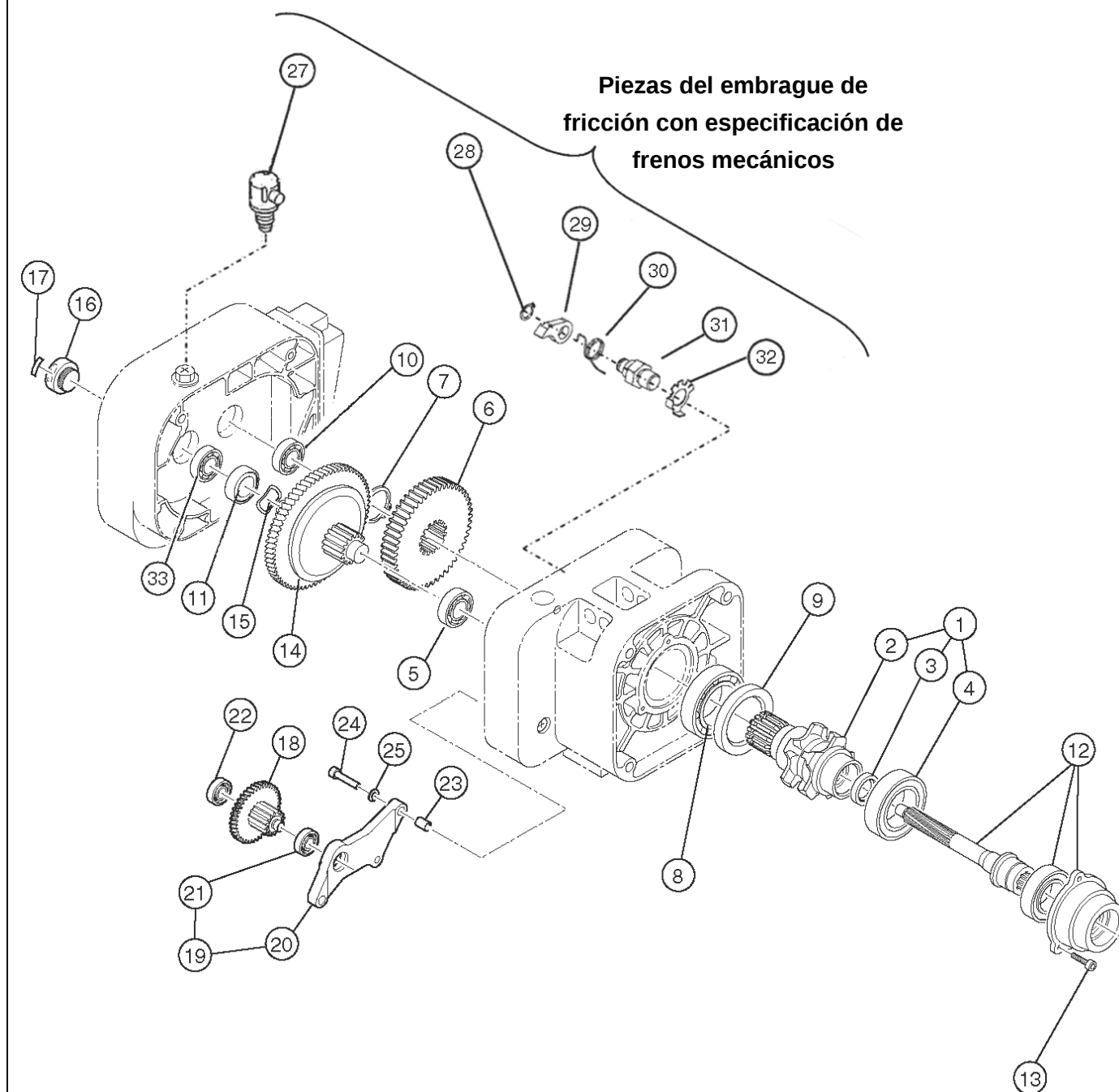
Figura 2-2 Partes del engrane
