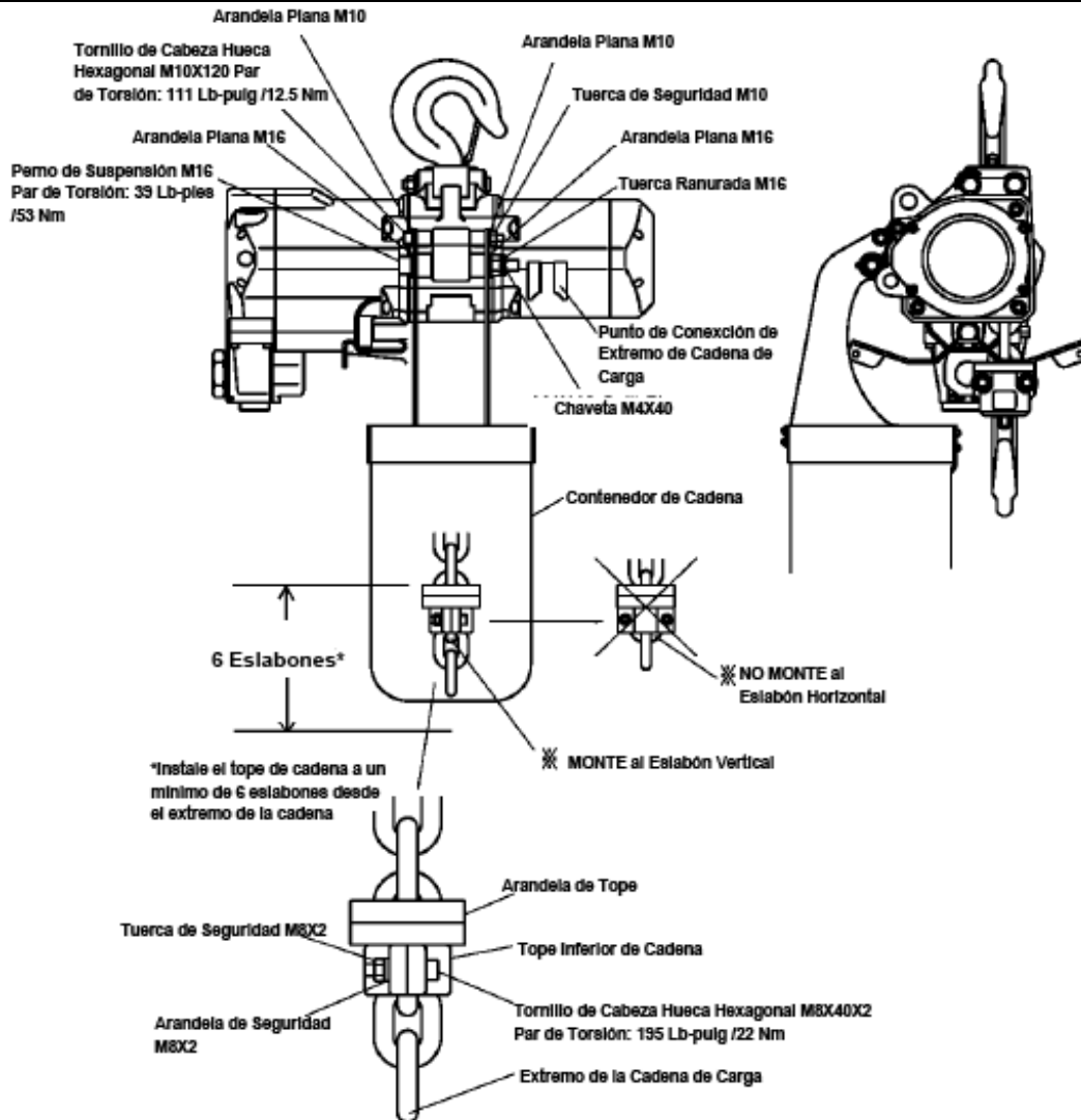
Figura 3-7 Instalación Opcional del Contenedor de Cadena
