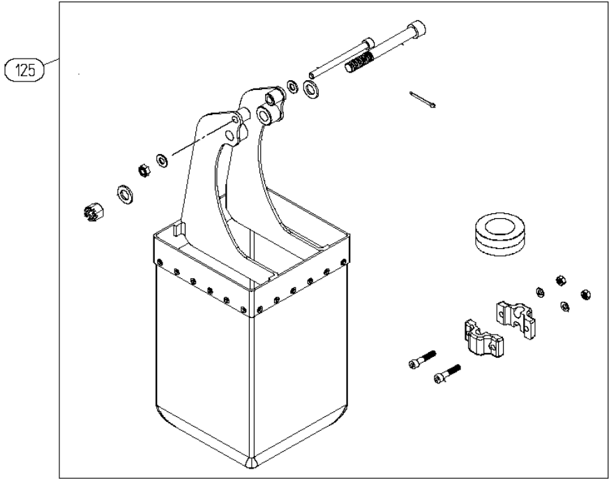
Figura 10-3 Ensamblaje del Contenedor de Cadena (Opcional)
