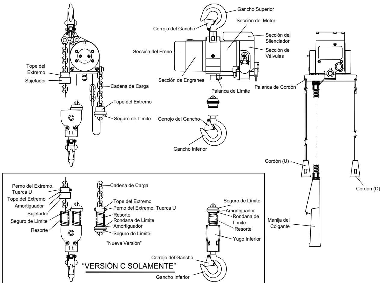
Figura 2-4 Diagramas de identificación de partes de los polipastos/tecle de cadena TCR 1000P2, 1000C2, 2000P2, 2000C2
