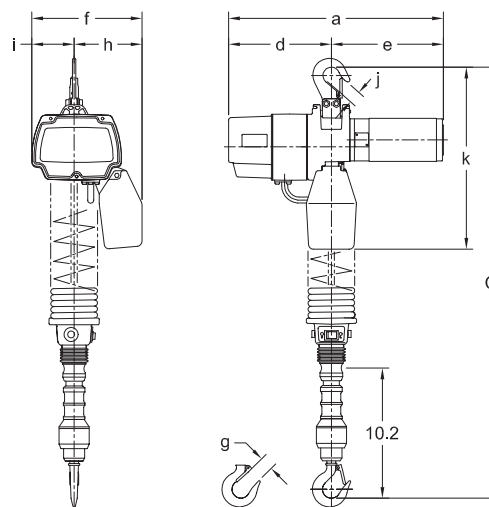
Modelo DA (dimensiones en pulgadas).
