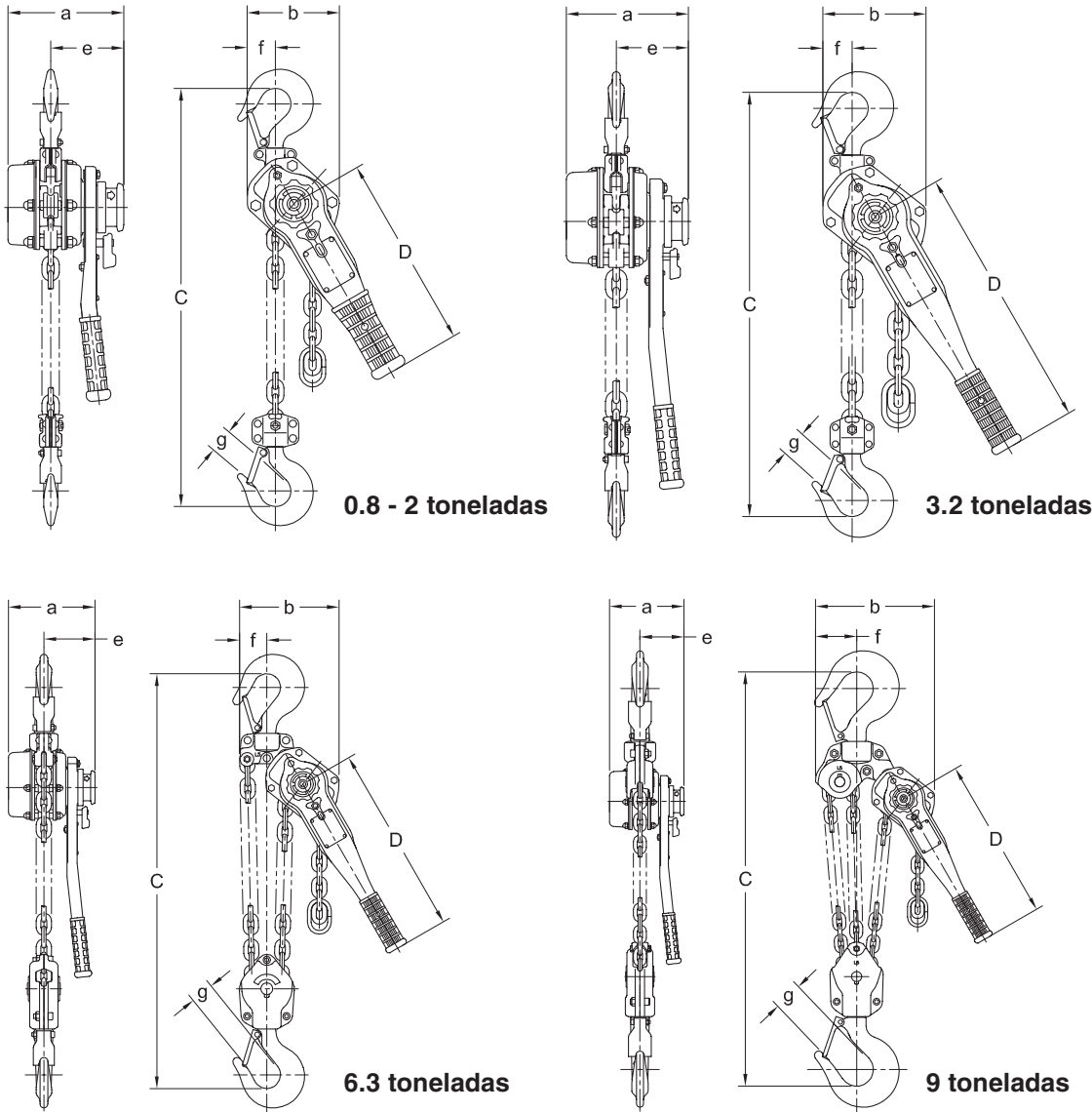
Polipasto/tecle de palanca LB
