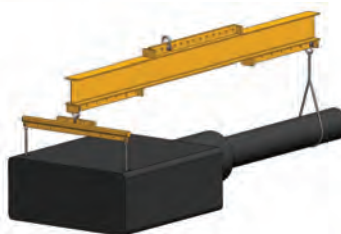
Sistema de izaje de tres puntos
