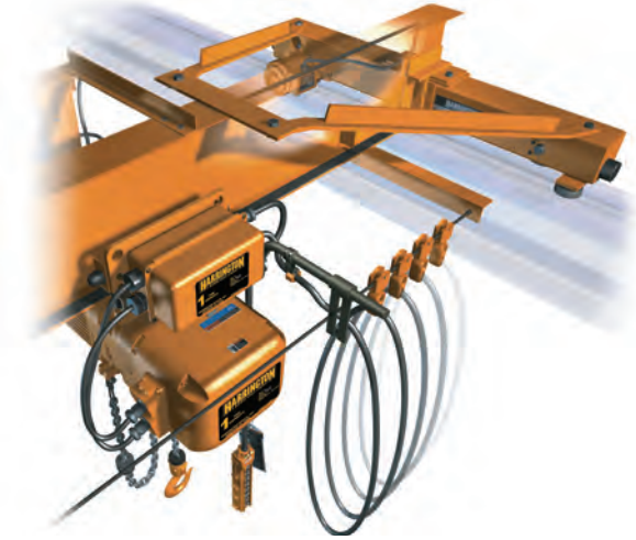
Grúas completas de alta resistencia, Clase C, con una viga, serie 3, aéreas
