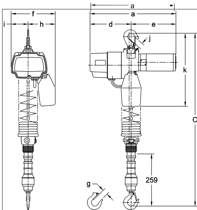
Figura 2-2 Dimensión del polipasto en los modelos DA (Consulte la Tabla 2-3)
