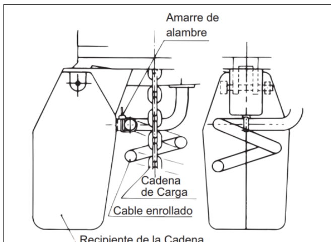
Figura 3-5 Diagrama para la instalación del cable del botón de presión tipo cilindro
