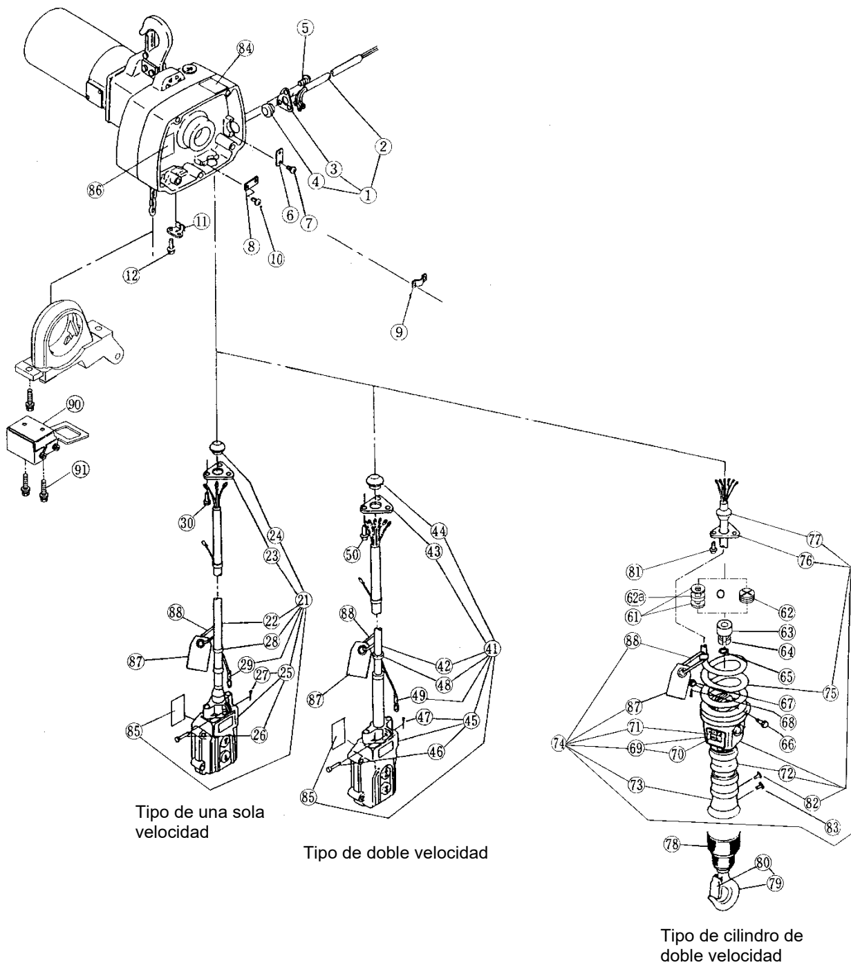
Figura 9-2 Partes del suministro de energía y colgante
